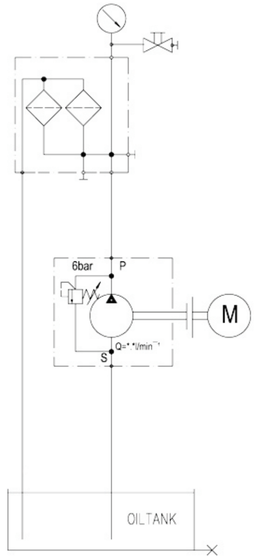
Fig. 2: Zeichnung OLU1D
