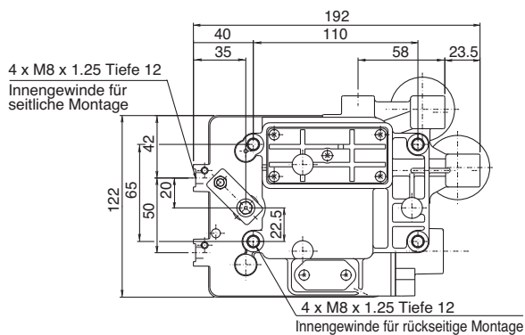
ANSICHT A
