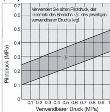
Diagramm ① Betriebsdruck - Pilotdruck (N.O.)
